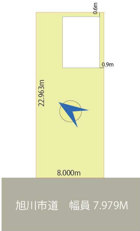
地籍図
